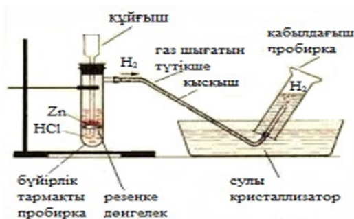
1-сурет – Сутекті суды ығыстыру әдісімен жинау
