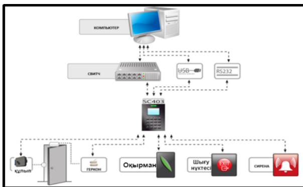
3-сурет – Кіргізу-шығару жүйесінің моделі
